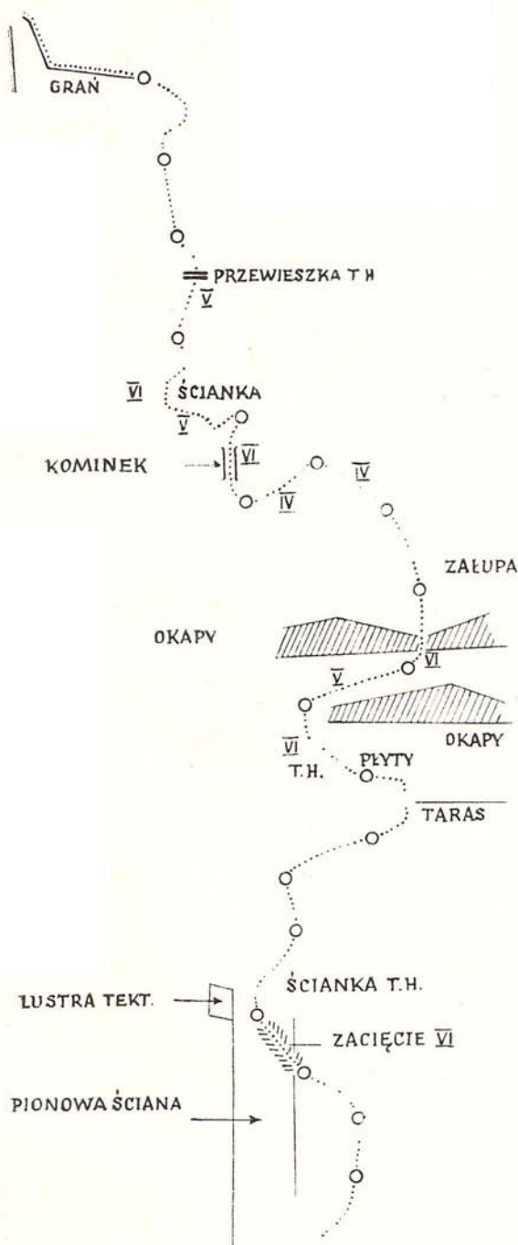
Schemat drogi wsch. ścianą Młynarczyka Rys. Józef Nyka
